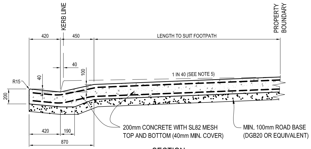
SECTION N. T. S.
